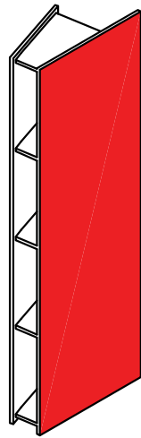
Torre de Satélite 2 57.5 x 180 x 27.5 cms
